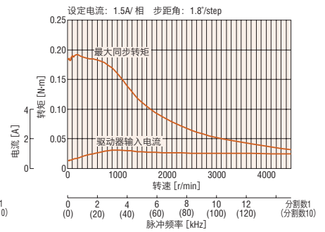
CVK225AK/CVK225BK
