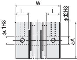
外形图
